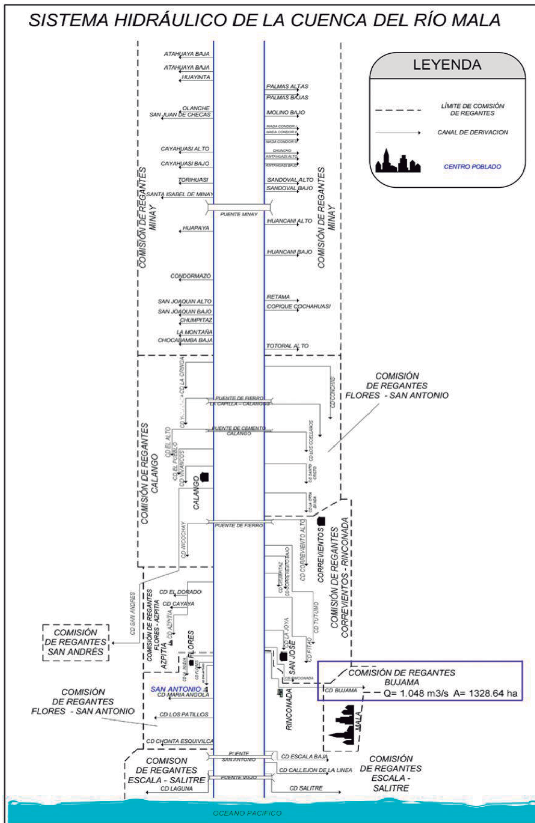
Figura 33. Esquema hidráulico de la cuenca del río Mala
