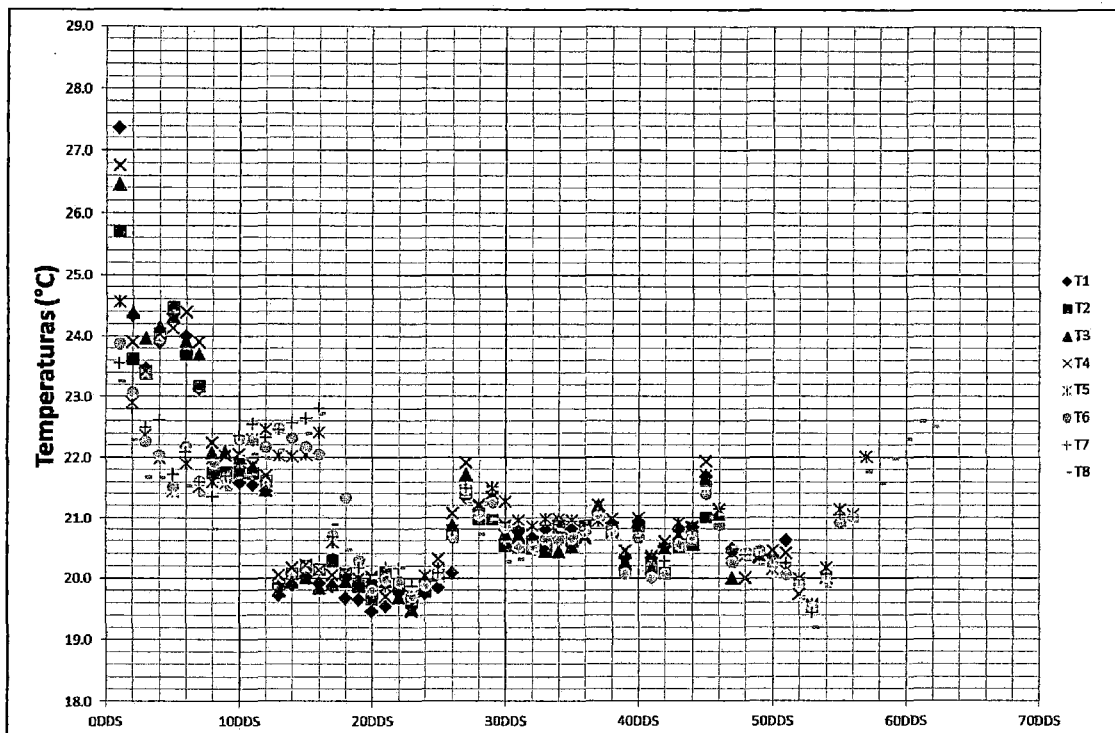
Figura 29: Temperaturas internas de las unidades experimentales en sus etapas de incubación e inducción-fructificación en todo el proceso productivo de los cuatro aislamientos de P. ostreatus cultivados en restos de cosecha.
